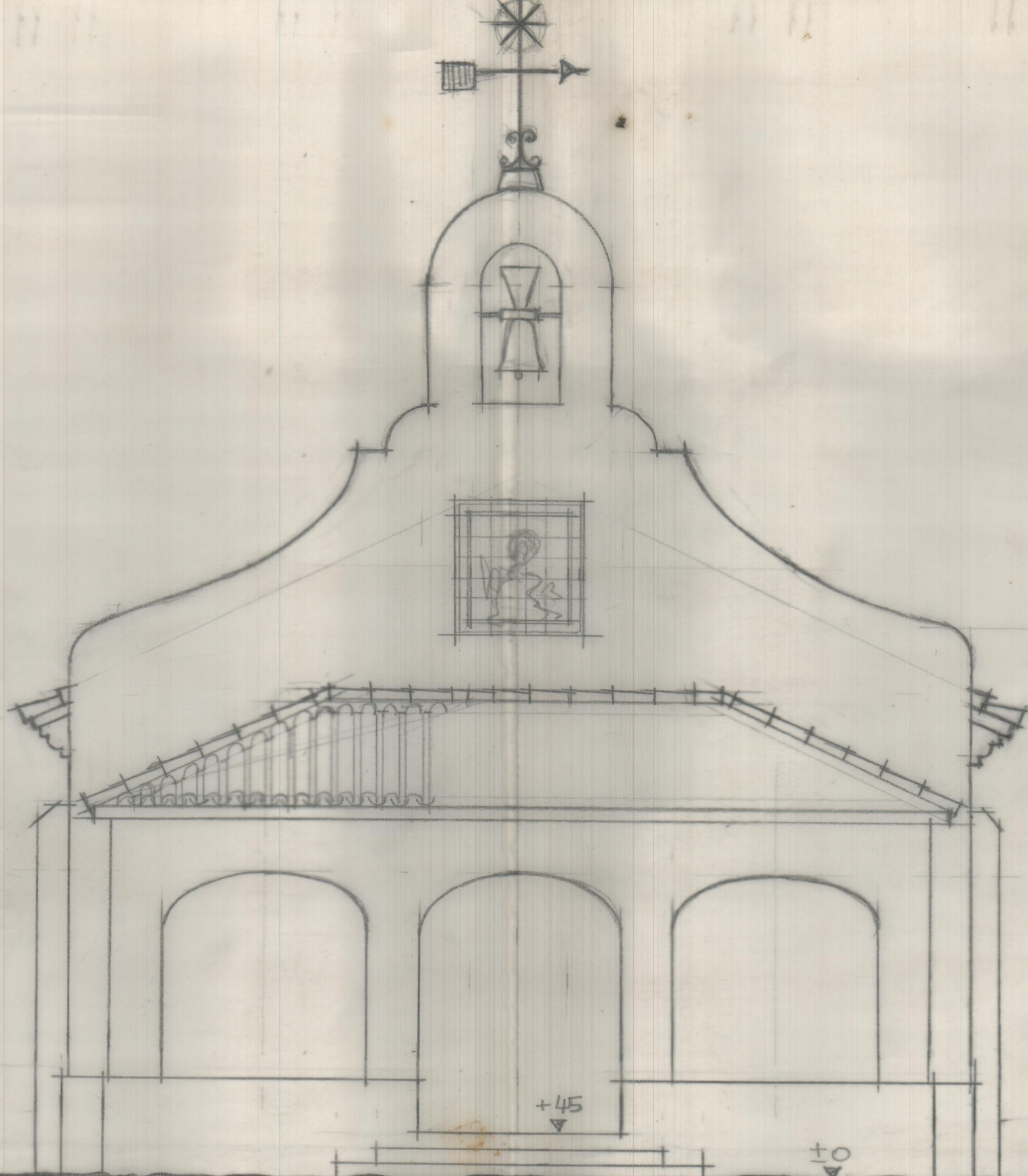
FRONTAL ESC = 1:50.
