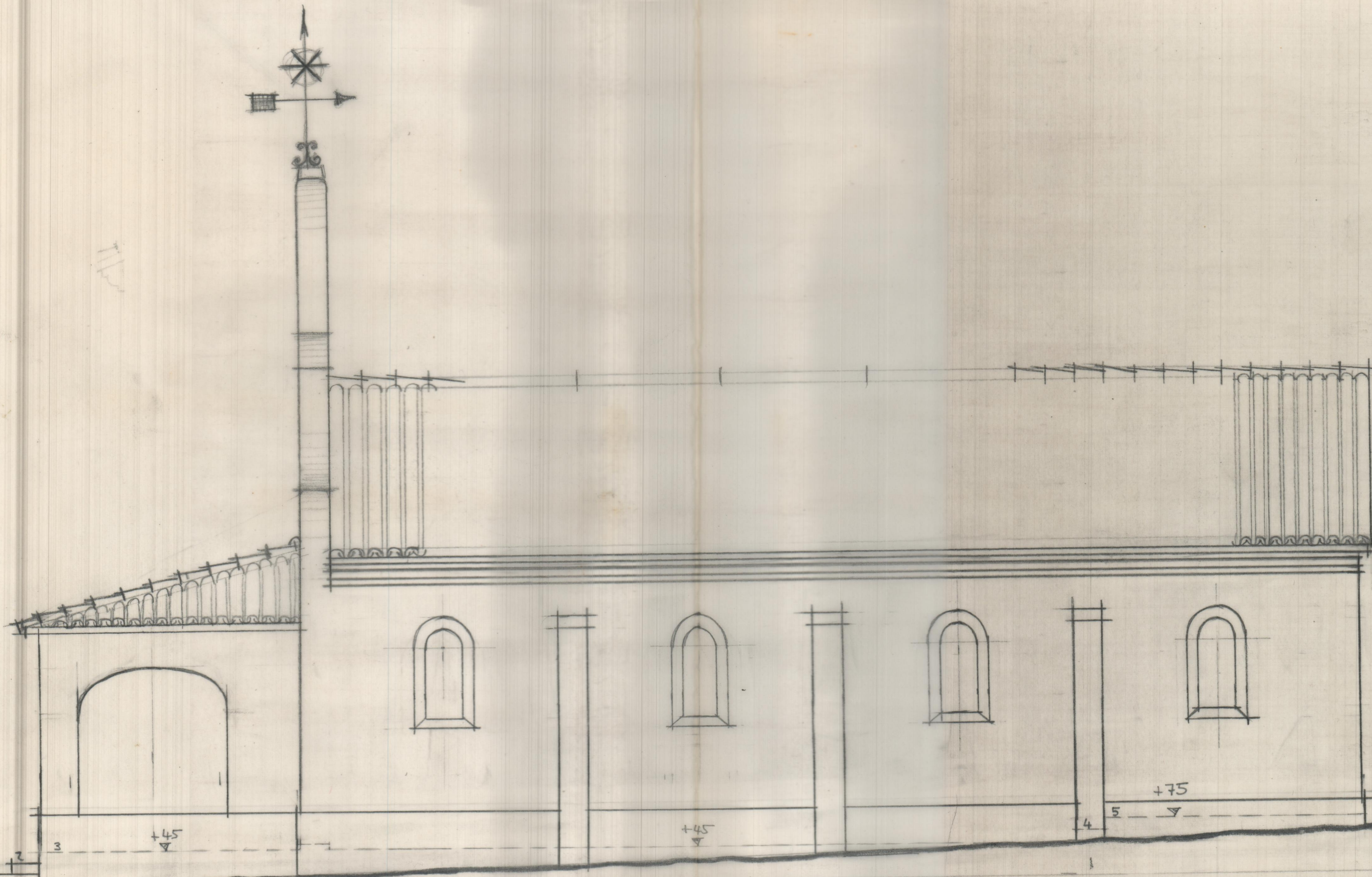
LATERAL. ESC. = 1:50.
