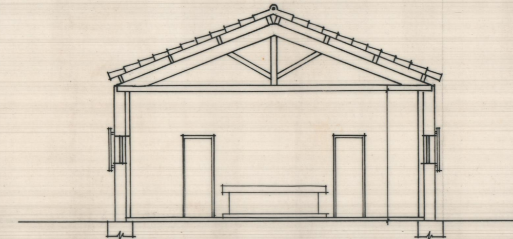
SECCIÓN A-B
