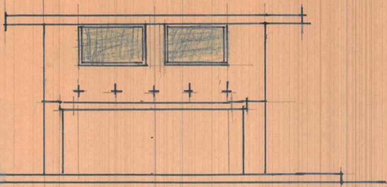
FRENTE
