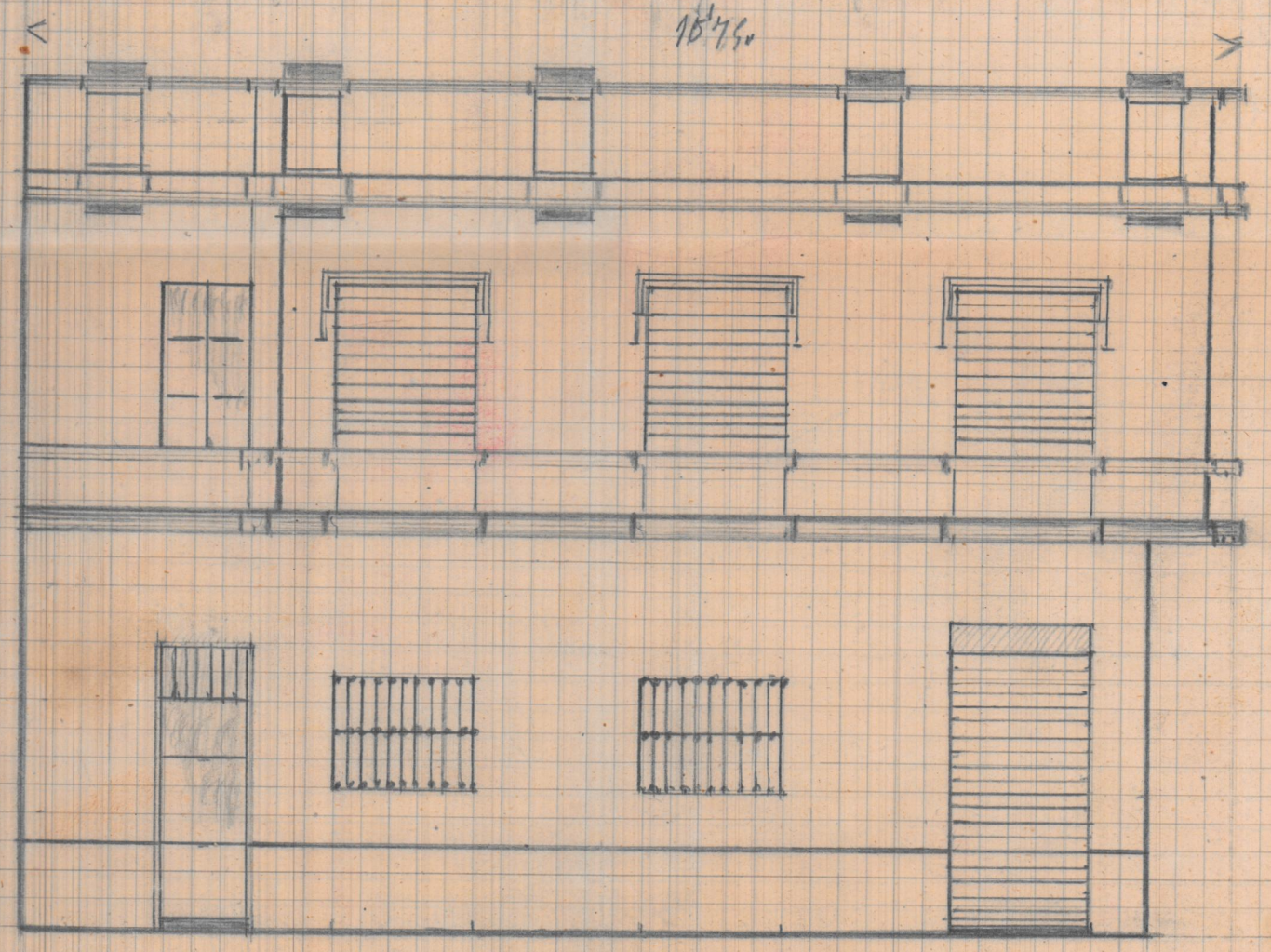
fachada de la fábrica de Industria Numero 27.
