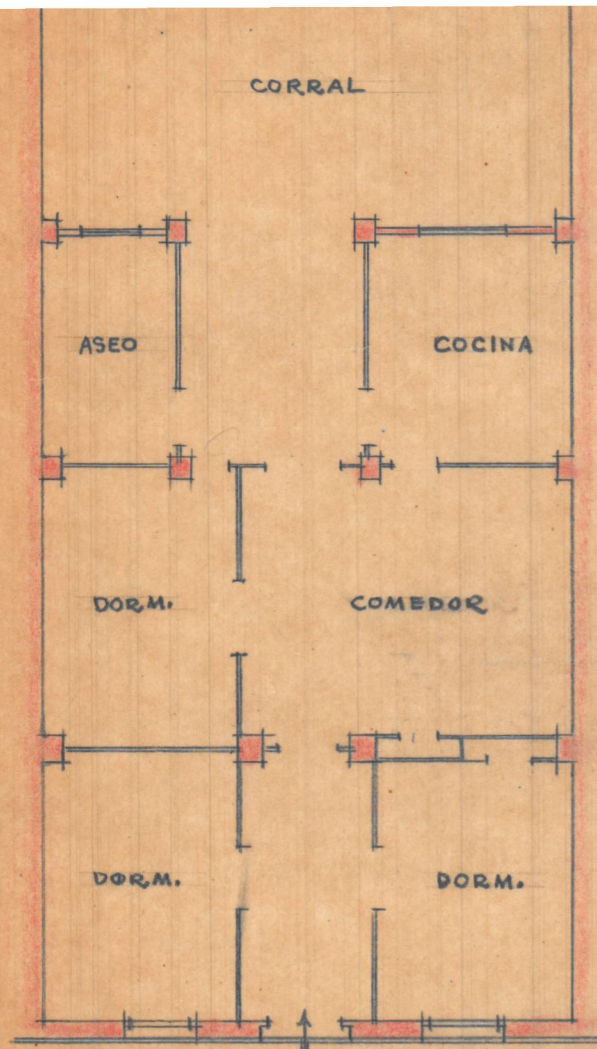
Planta
