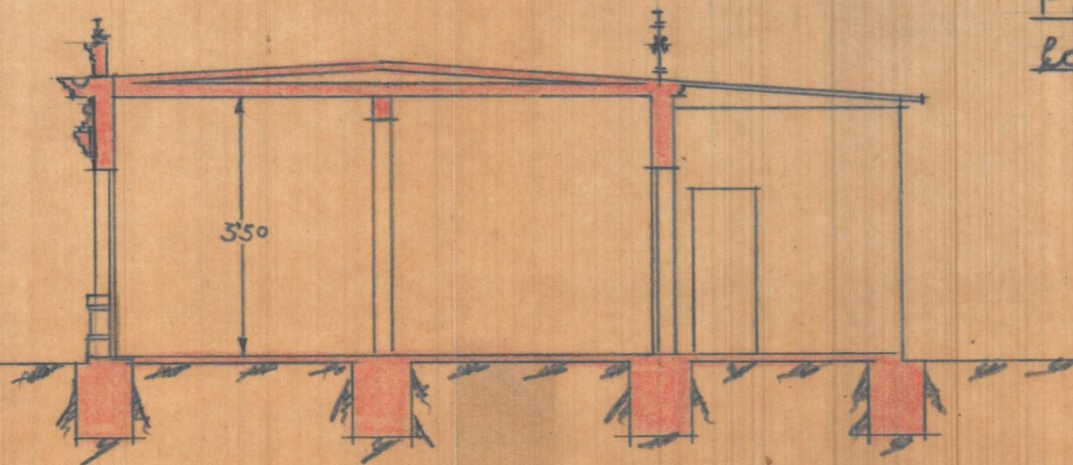
Sección
