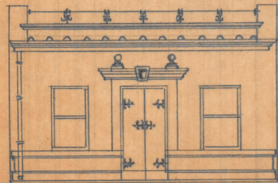
Fachada
