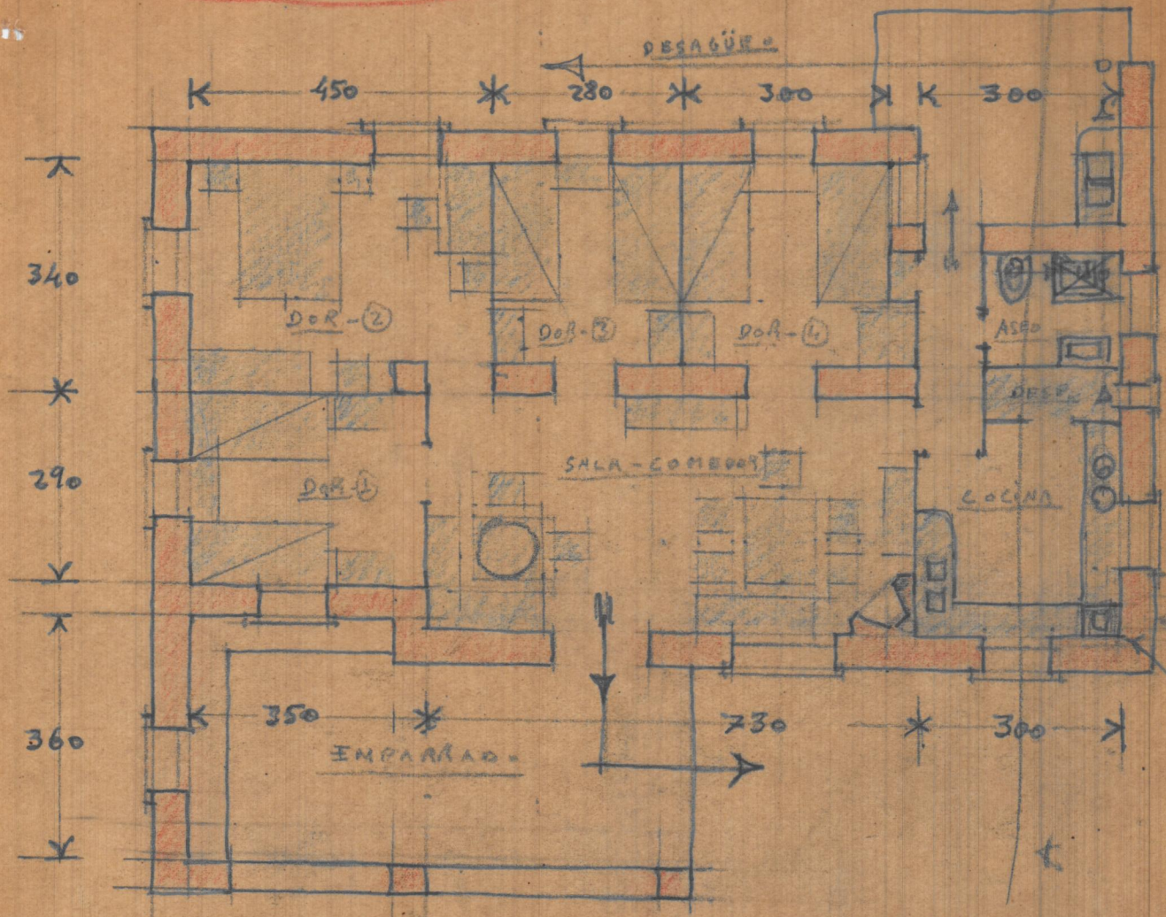
PLANTA DE DISPOSICION
