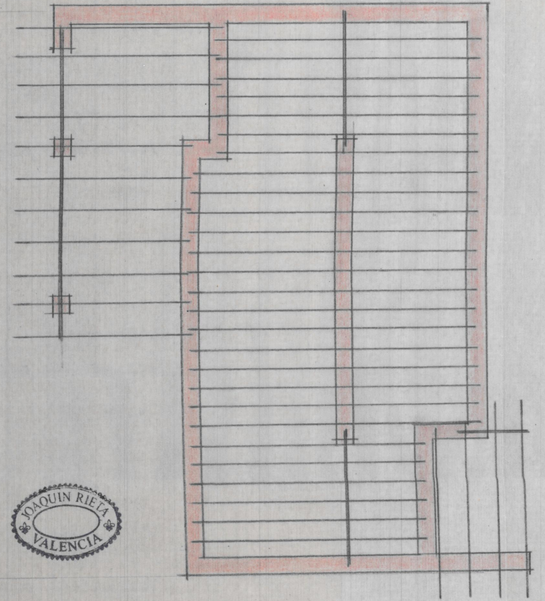
Planta de entramados
