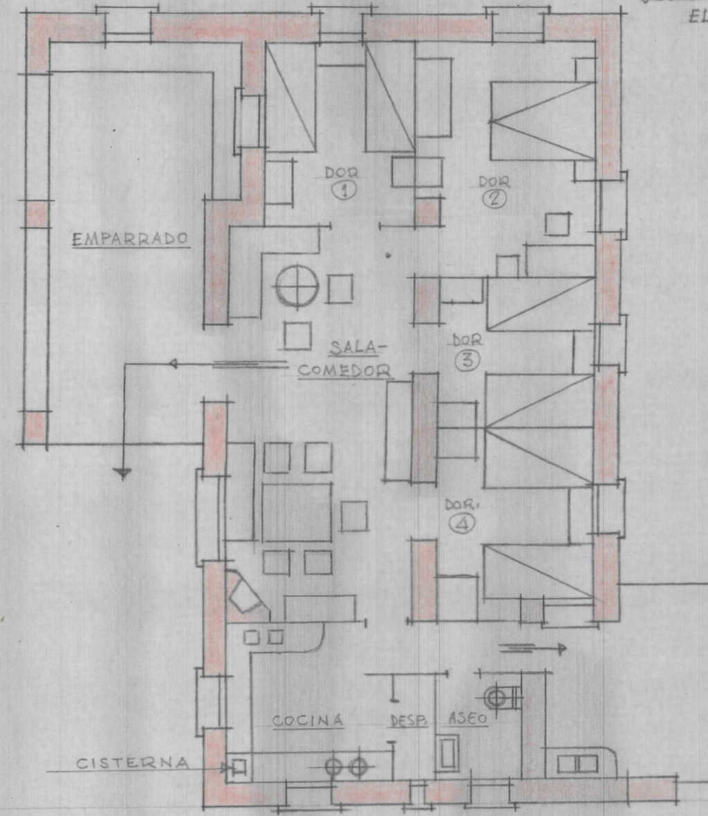
Planta de distribución
