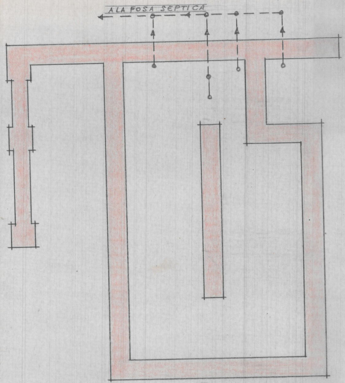
Planta de cimientos y de daques
