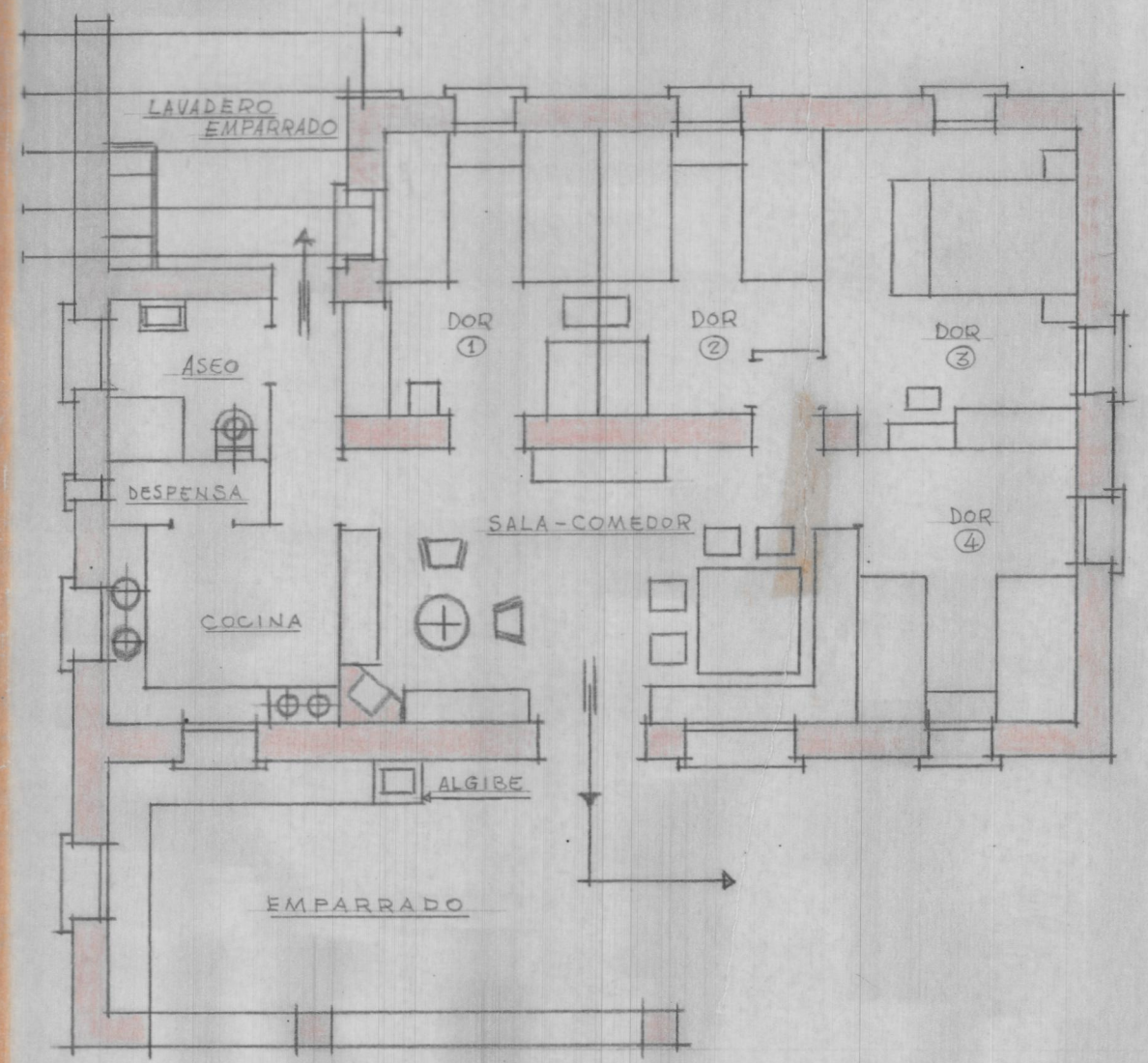
Planta de disposicion
