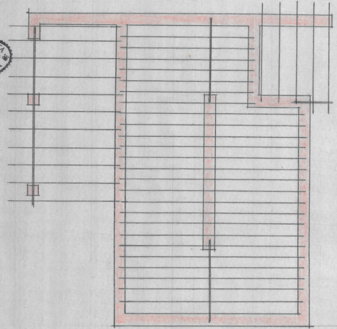
Planta de entramados
