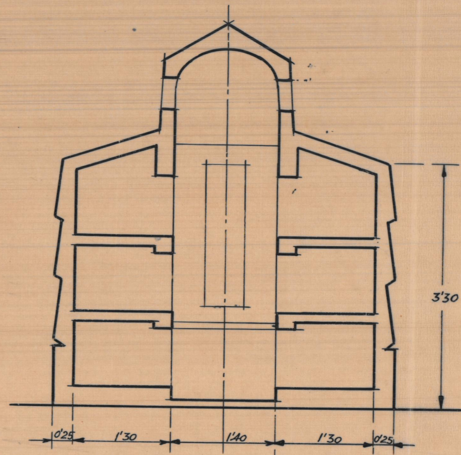
Sección A-B
