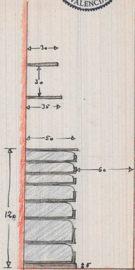
SECCION CD
