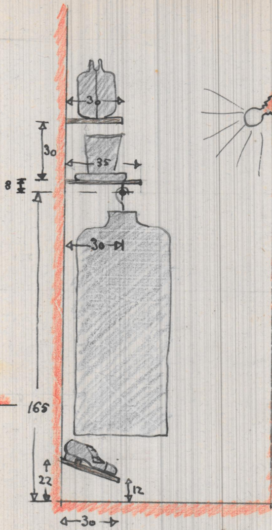
SECCION AB
