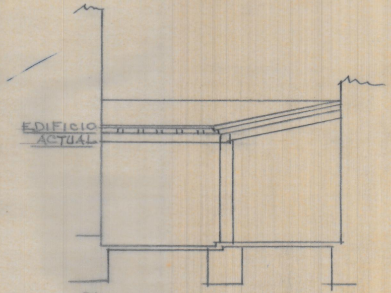
Sección AB
