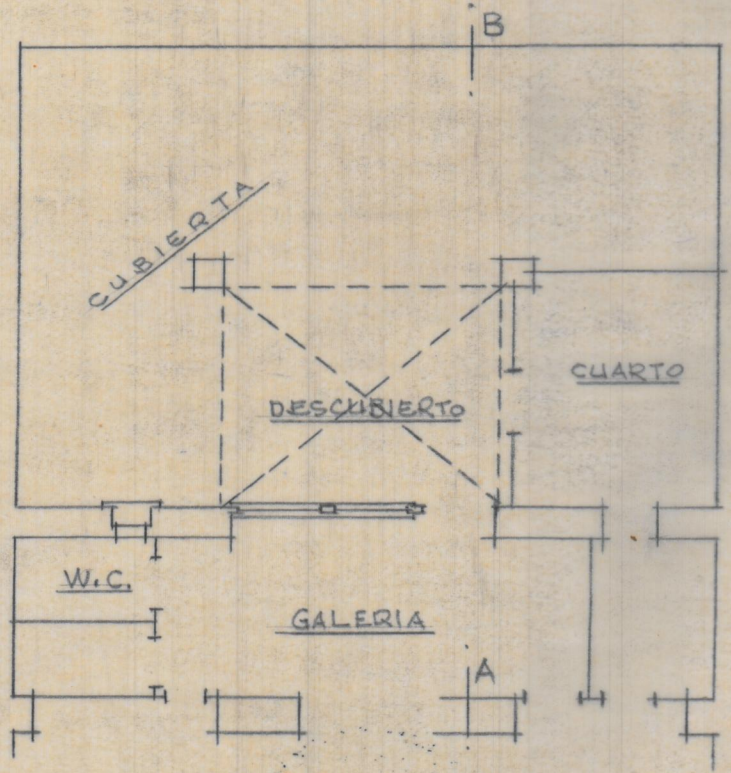
Planta de disposición
