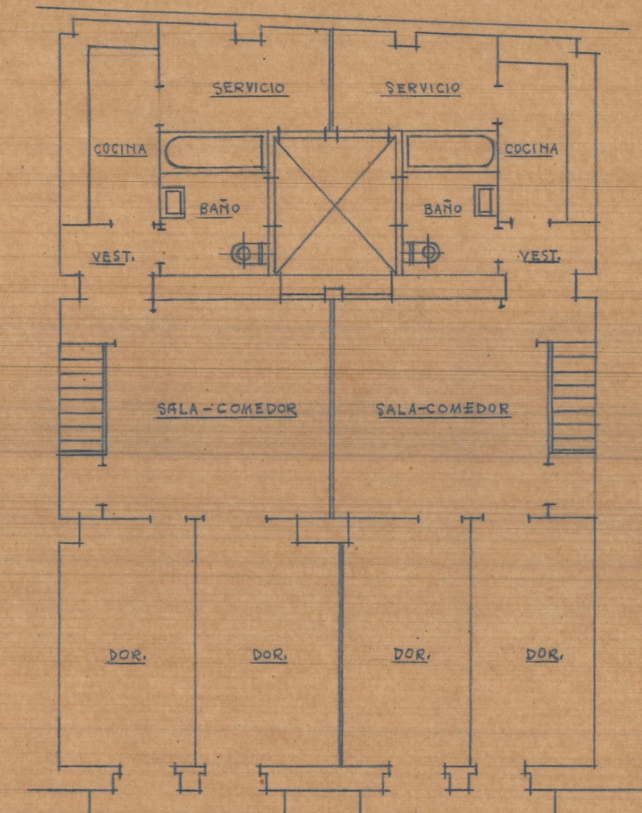
Nuevo piso - PLANTA -
