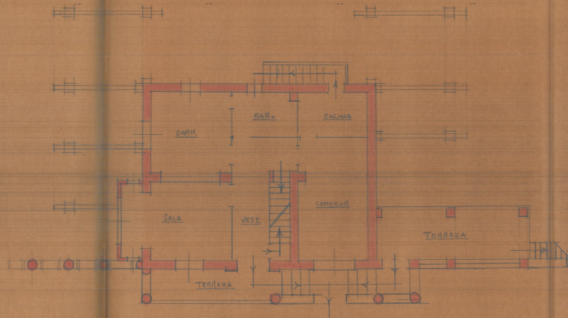
PLANTA PRINCIPAL
