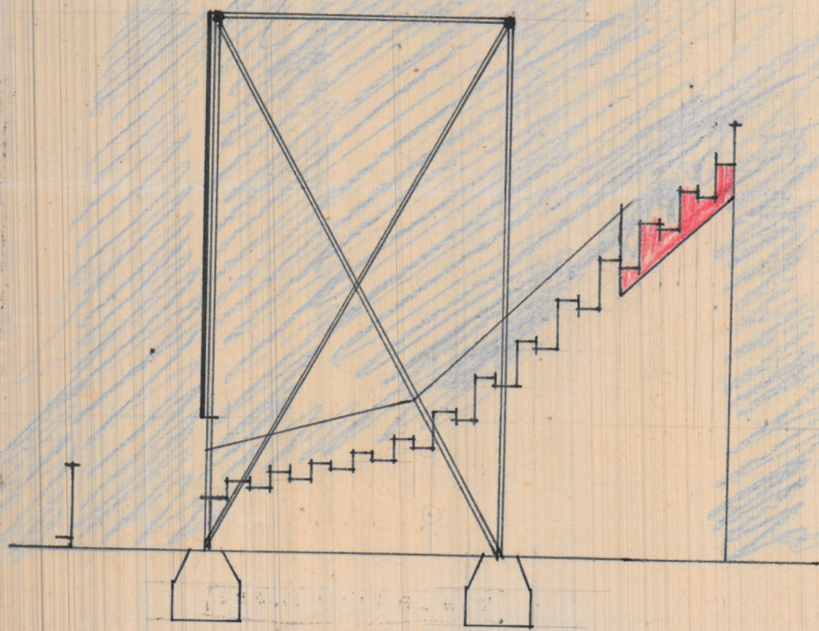
PANTALLA SECCION C-D
