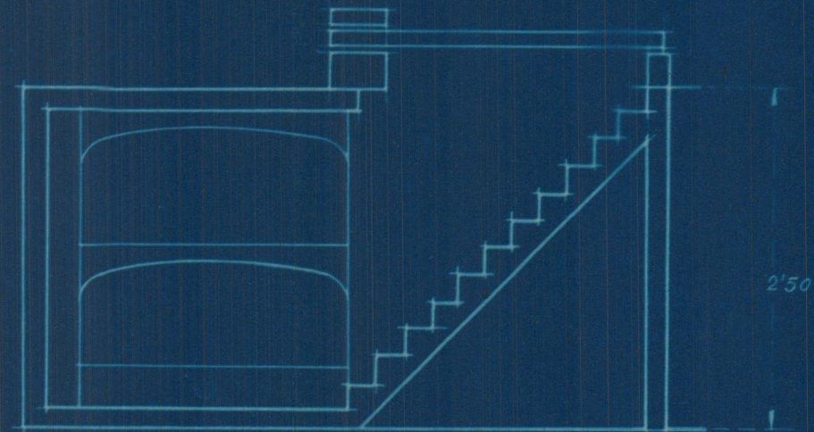
Sección longitudinal
