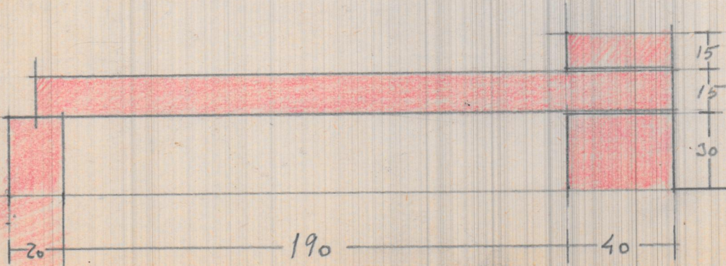
Sección longitudinal
