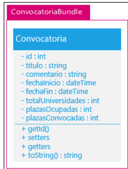
Figura 29 - Diagrama de clases Convocatoria
