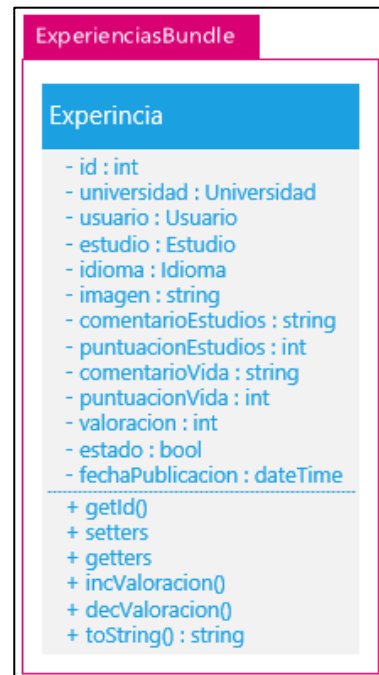
Figura 31 - Diagrama de clases Experiencias
