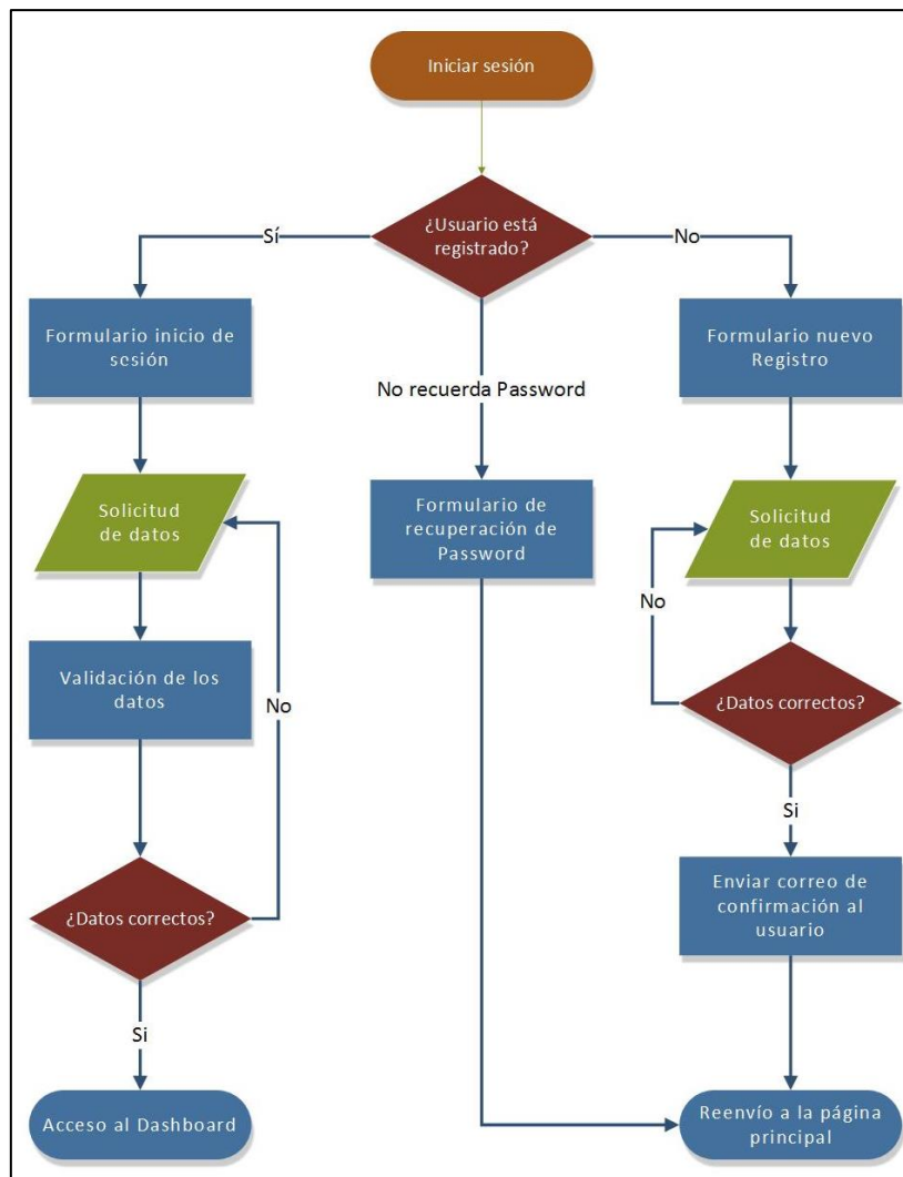
Figura 36 - Diagrama de flujos login/registro
