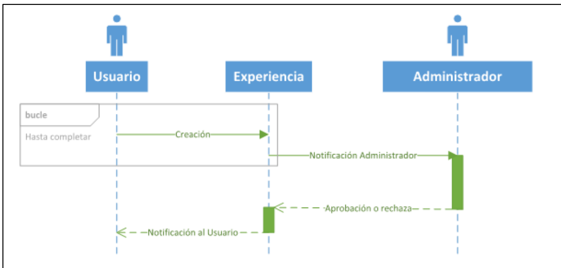
Figura 38 - Diagrama de secuencias de la aprobación de una experiencia
