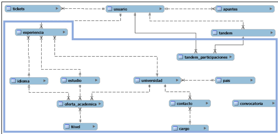
Figura 32 - Diagrama de Bases de Datos
