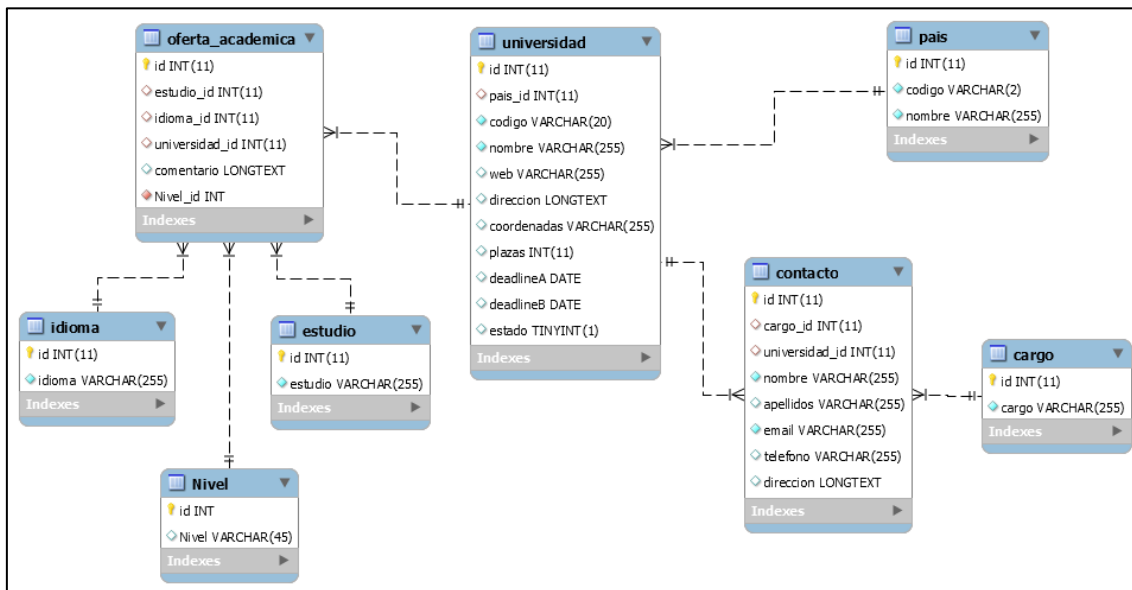
Figura 41 - Diagrama ER de universidades, contactos y oferta académica
