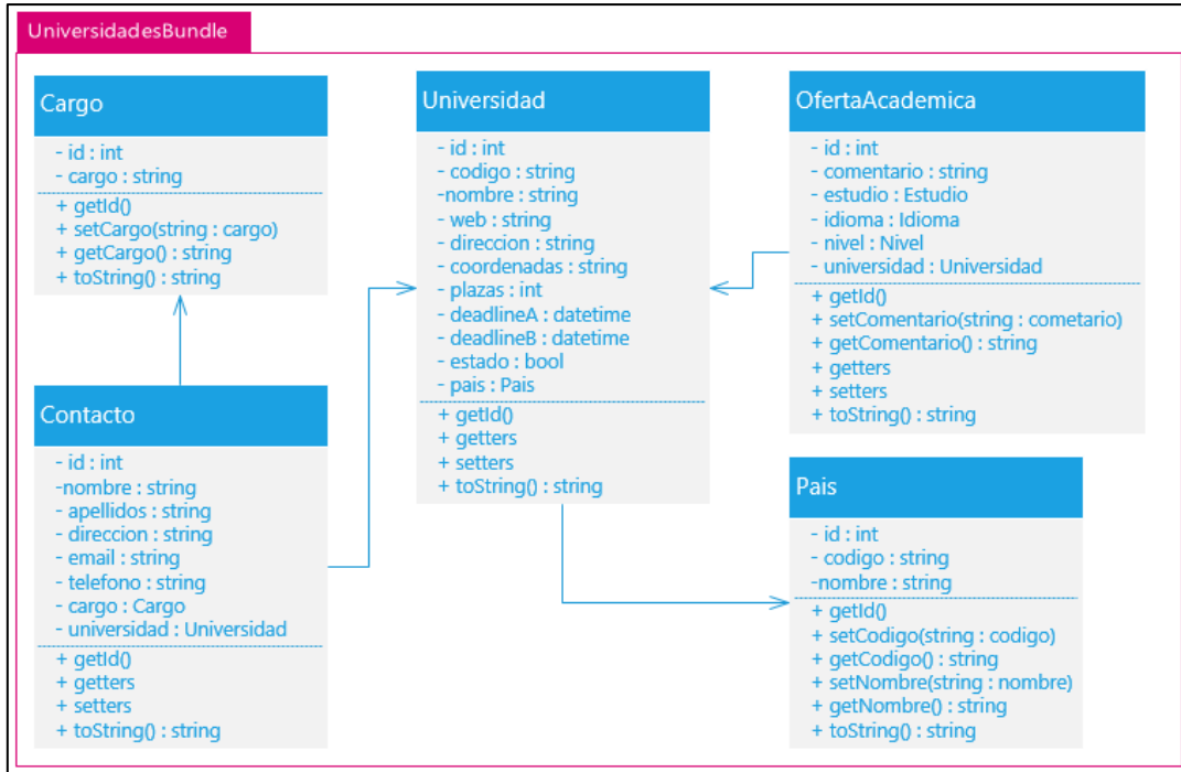
Figura 30 - Diagrama de clases de Universidades
