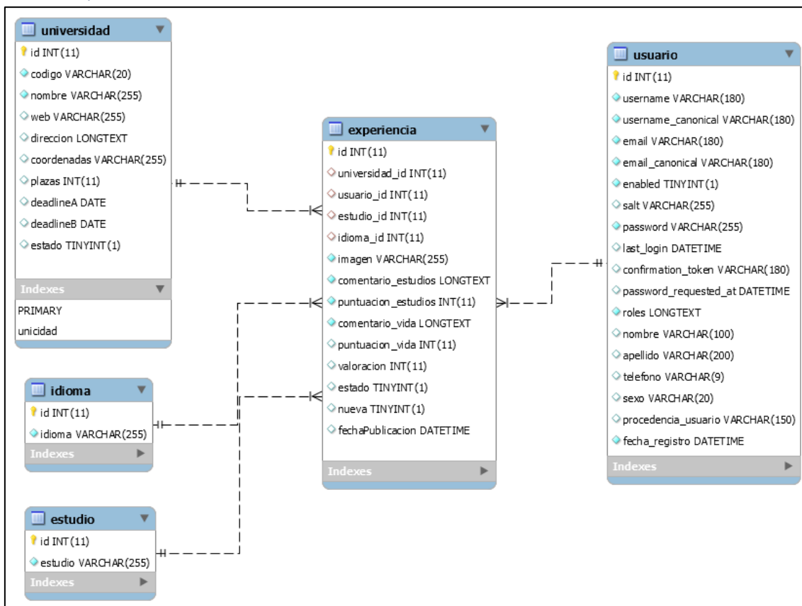
Figura 40 - Diagrama ER de experiencias Erasmus
