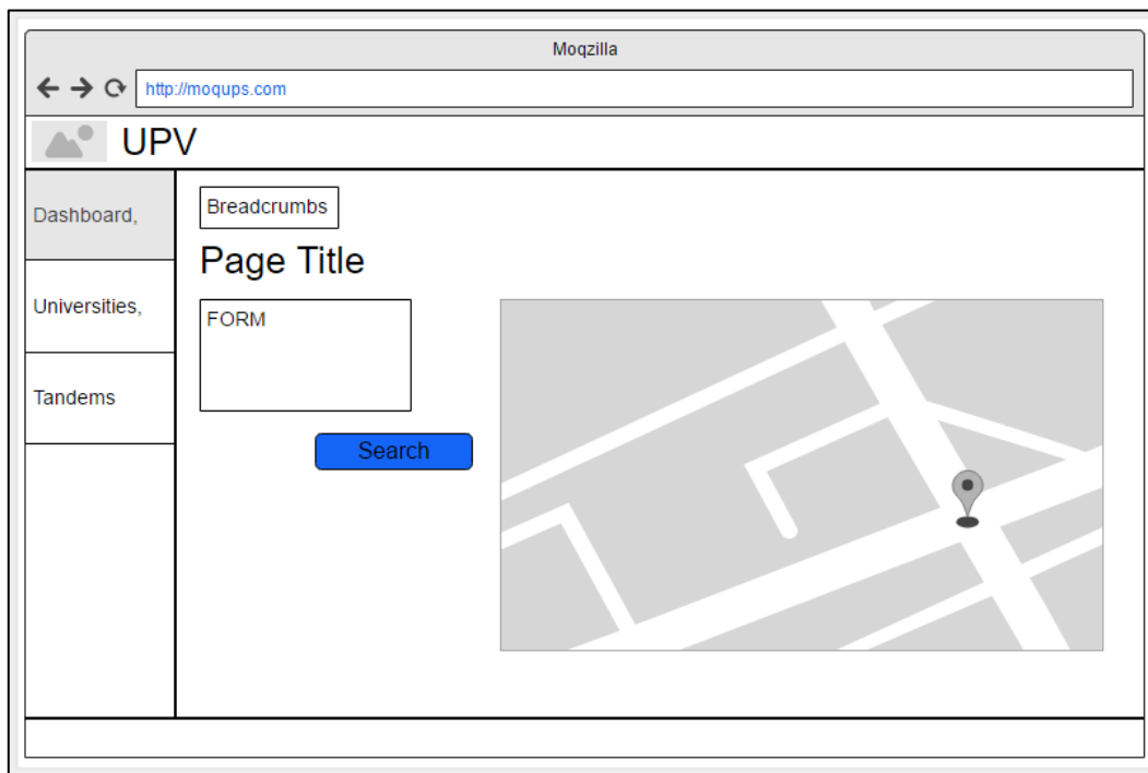
Figura 35 - Boceto del módulo de búsqueda de destinos Erasmus
