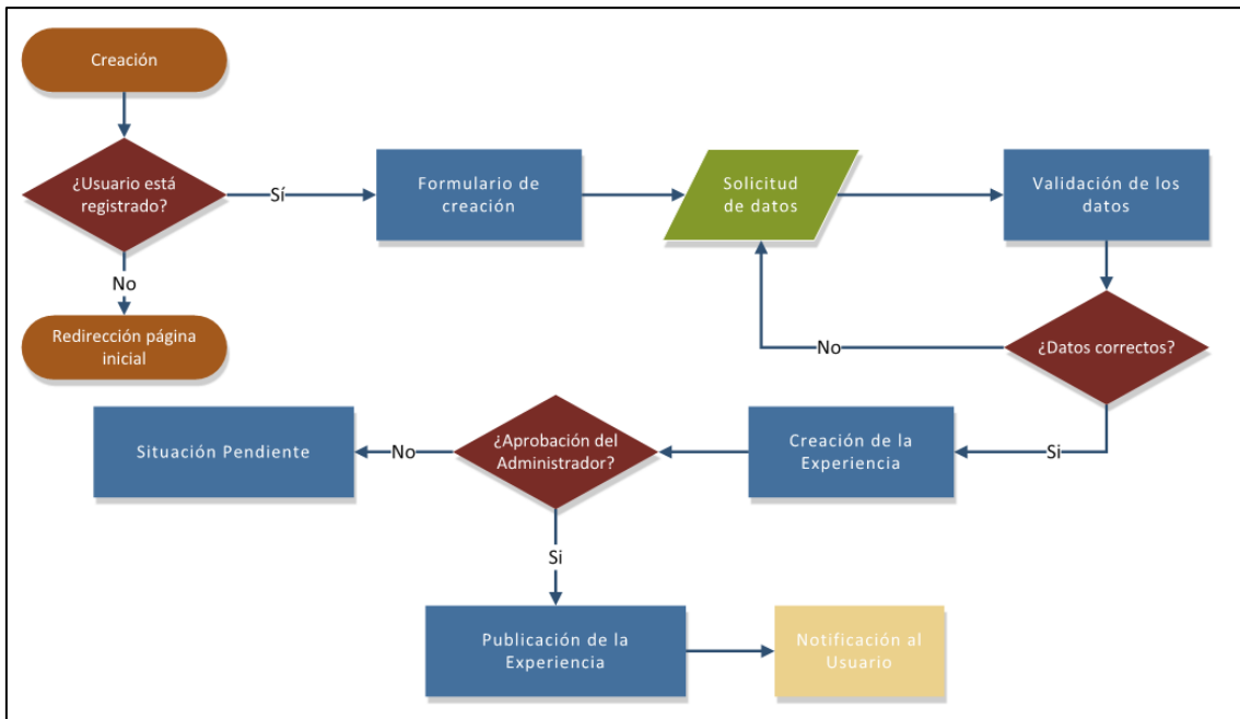
Figura 37 - Diagrama de flujos de creación de una experiencia
