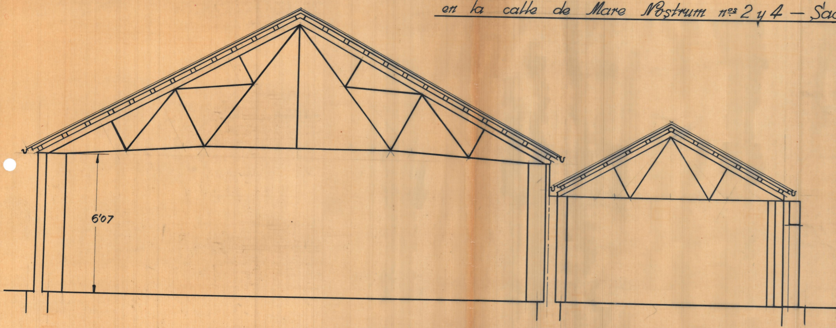
Seccion A-B
