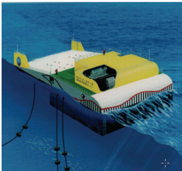
Figura 30: El Mighty Whale. ( www.textoscientificos.com/energia/dispositivos-generacion-energia-olas )
