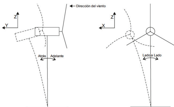
Figura 3: Grados de libertad de un gran generador eólico. (Suryanarayanan, and Dixit, 2005.)
