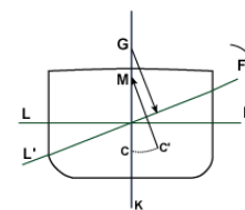
Figura 17a: Estabilidad en flotación
