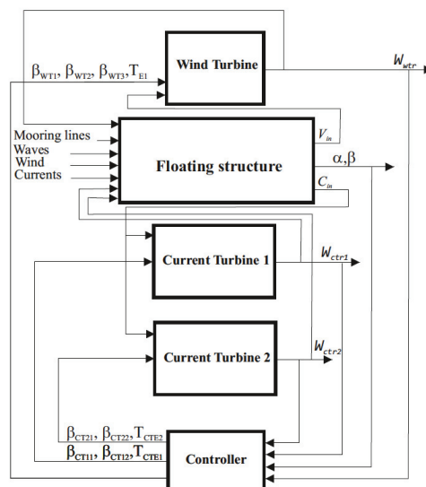
Figura 18: Diagrama de bloques del sistema de control integrado
