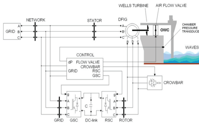
Figura 25: Esquema general del Sistema OWC. (Ormaza, 2012)
