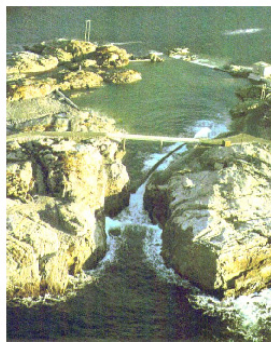
Figura 32: La planta Tapchan. ( www.textoscientificos.com/energia/dispositivos-generacion-energia-olas )
