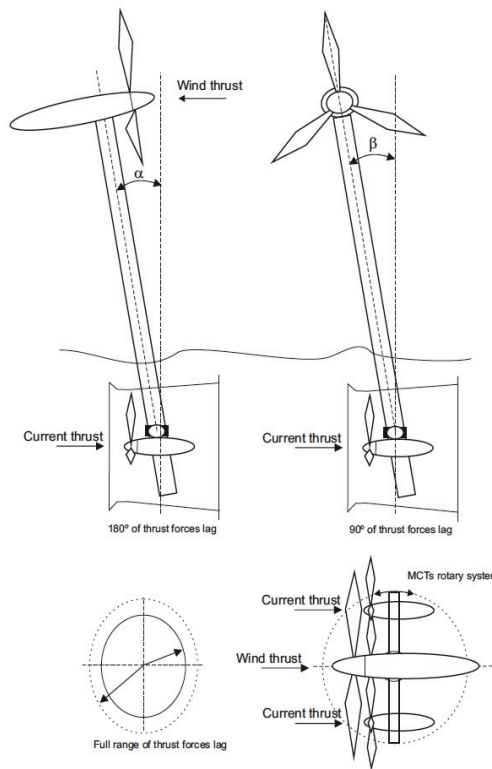
Figura 17b: El Módulo Integrado de Generación MICHEGER
