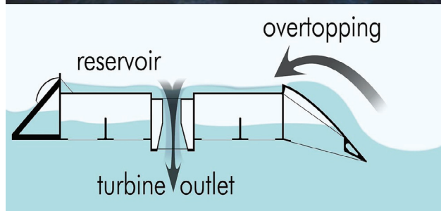
Figura 26: Disposición y funcionamiento del Wave Dragon. (Drew et al., 2009)
