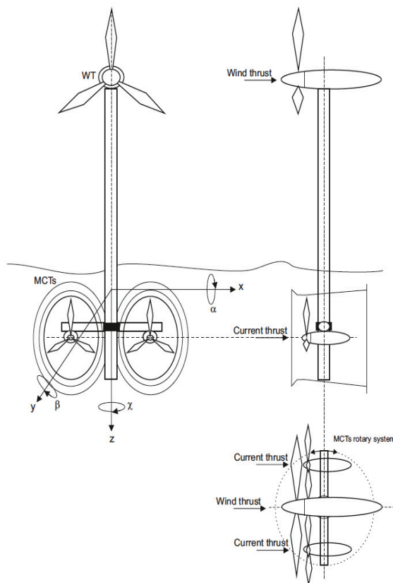
Figura 16: El Módulo Integrado de Generación MICHEGER
