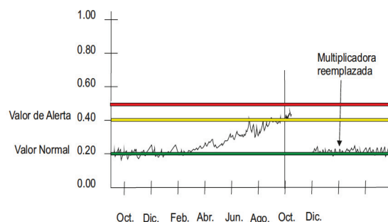
Figura 36: Análisis de tendencia de las vibraciones en una multiplicadora
