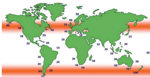
Figura 19: Distribución mundial de Kw/m frente de ola. (Comission, E. Ocean energy conversion in Europe, 2006)
