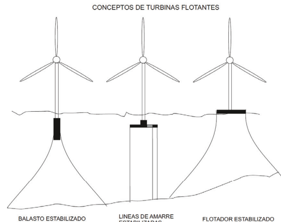
Figura 1: Propuestas principales de estructuras flotantes. (Jonkman and Buhl, 2007)
