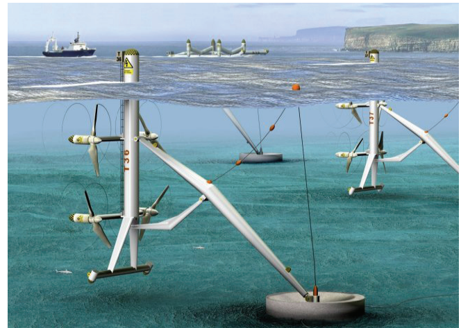
Figura 12: Diseño de emplazamiento de turbinas de flujo de 4MW en Pentland Firth a una profundidad de 60 metros y un rotor de 20 m para la generación de energía. (Ben Elghali et al., 2007)
