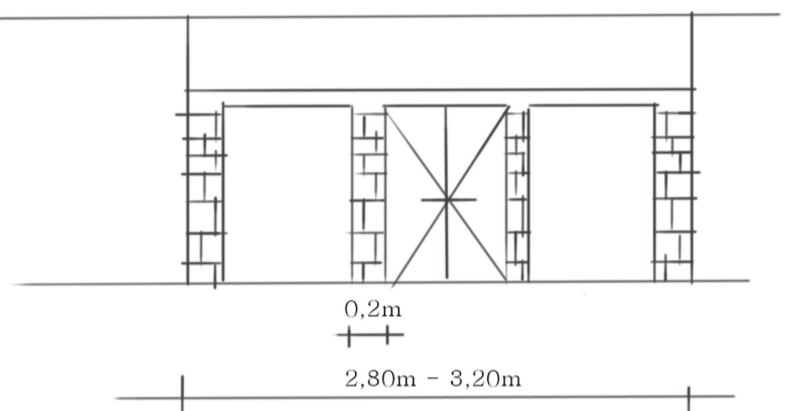
Tipo Fachada 3
