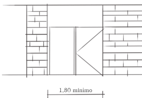
Tipo Fachada 1
