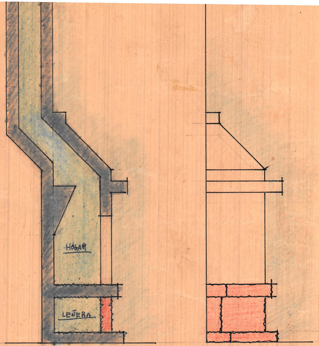
SECCION VERTICAL
