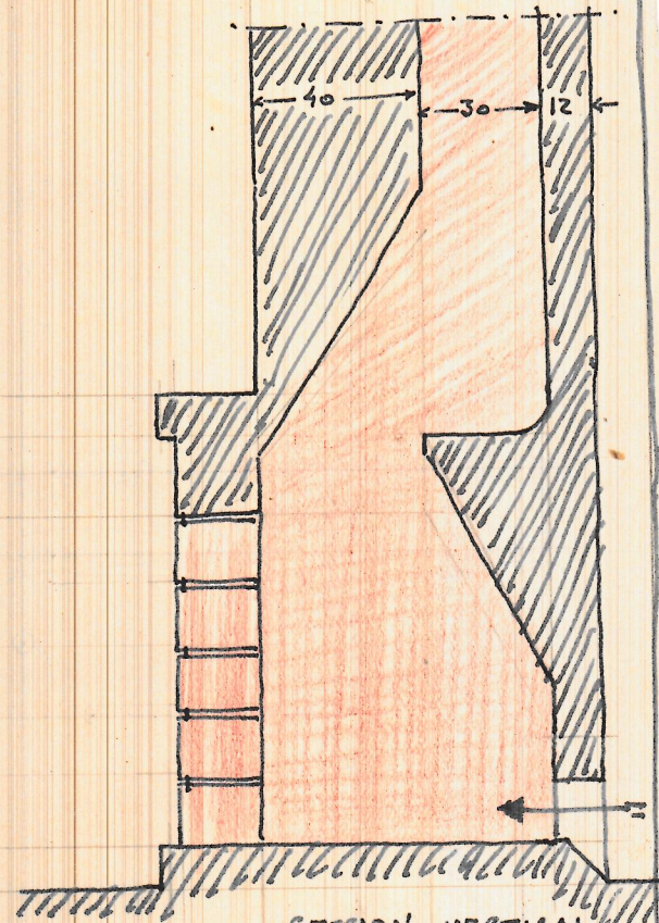
SECCION VERTICAL
