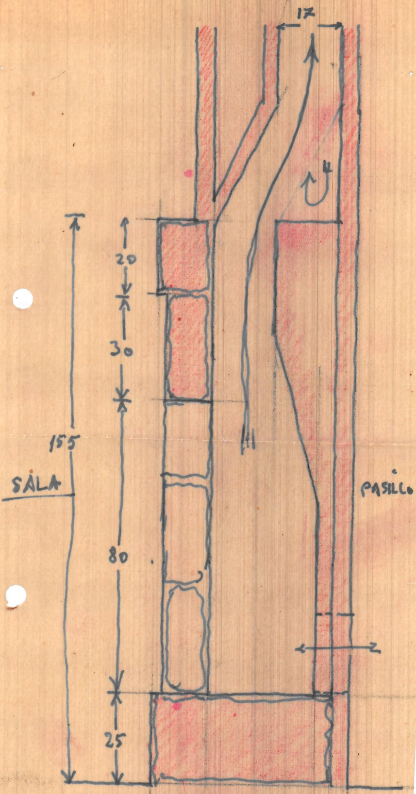
SECCION VERTICAL 5-1:10
