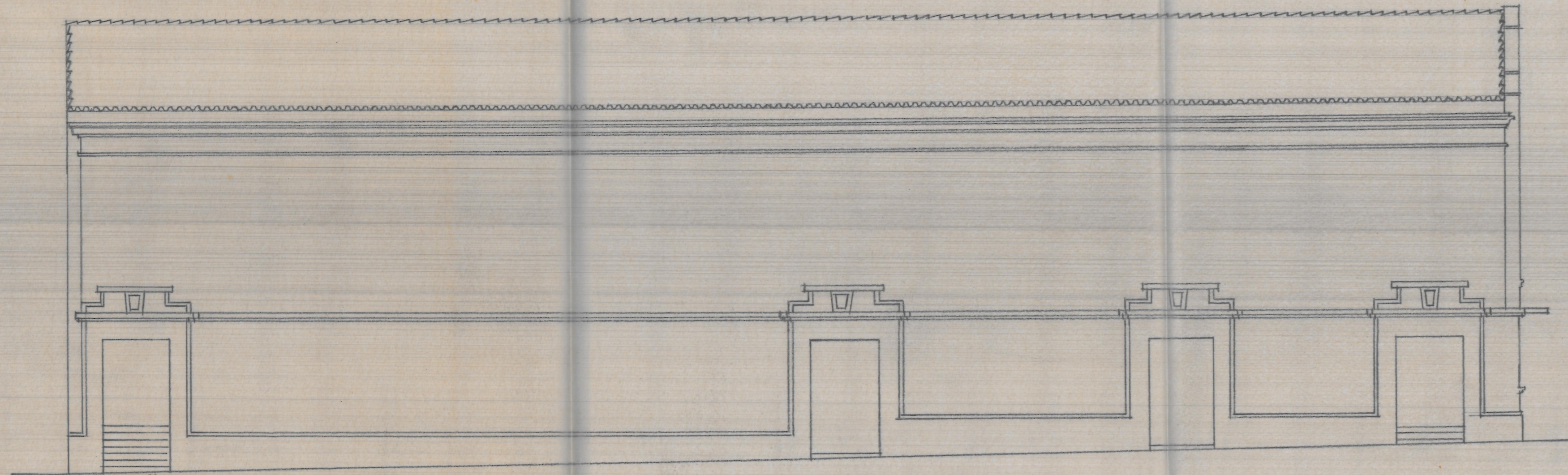
Fachada lateral
