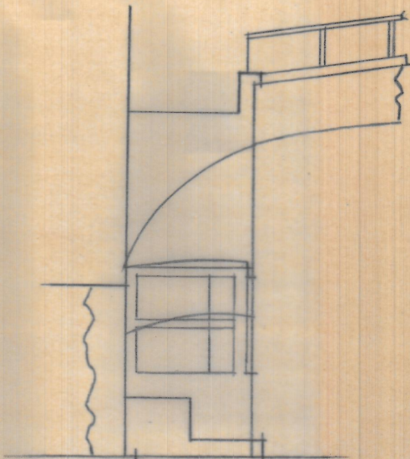
Sección vertical por A-B-C-D.
