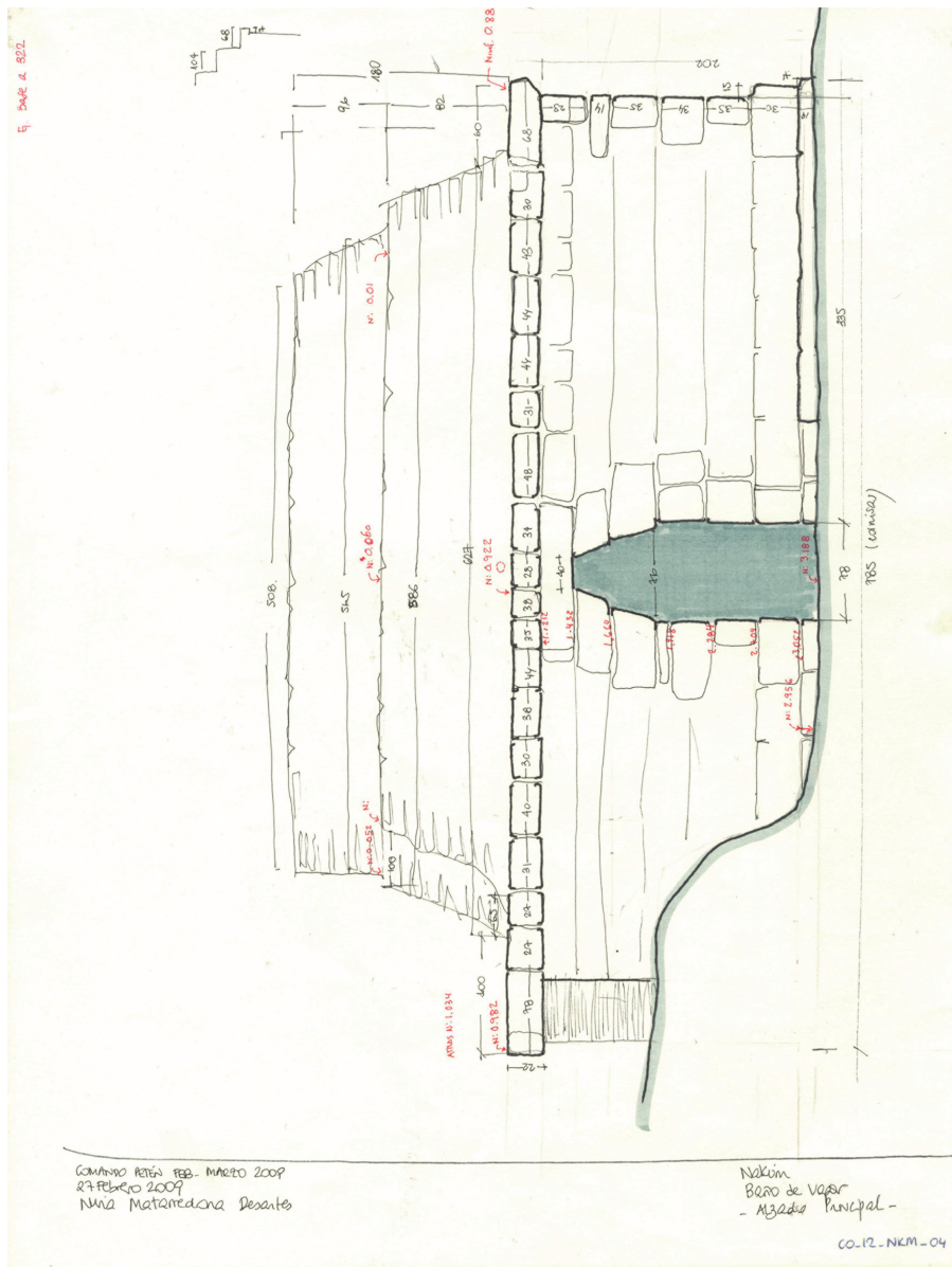
FIGURA 6. Croquis del alzado principal del temascal de Nakum (edificio 26). Dibujo de Nuria Matarrredona.
