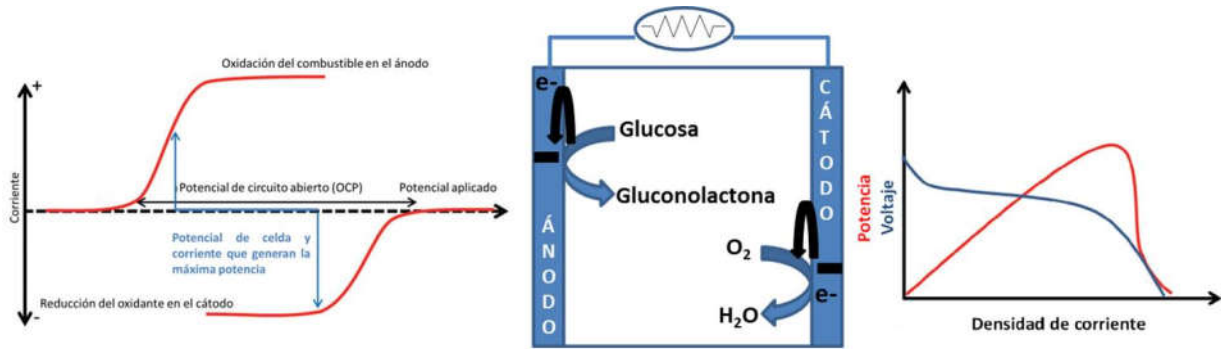
Fig. 2: Esquema general de funcionamiento de una biopila de glucosa.
