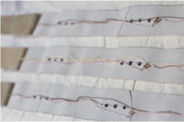
Fig. 5 Proceso de creación de las tiras luminosas. Vista de la electrónica interior, 2012.
