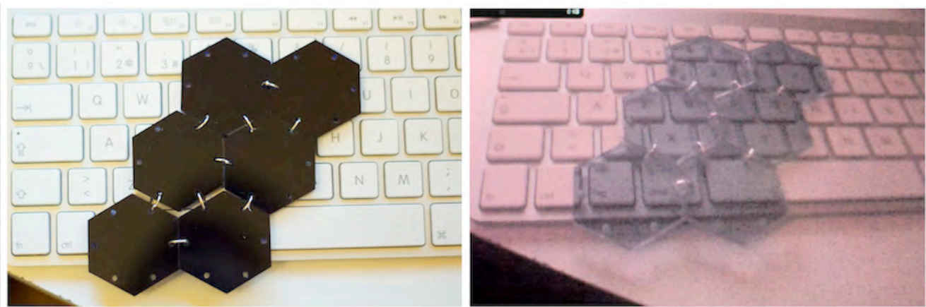
Fig. 2 Imagen a simple vista del material del vestido de percepción transparente al infrarrojo e imagen a través de la cámara de infrarrojos.
