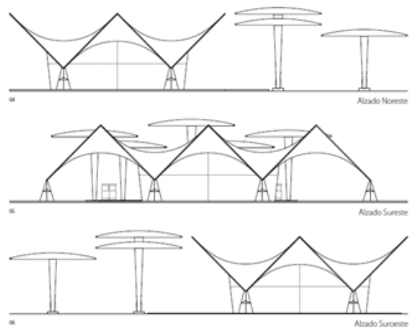
Figura 16. Alzados El Rebollet
