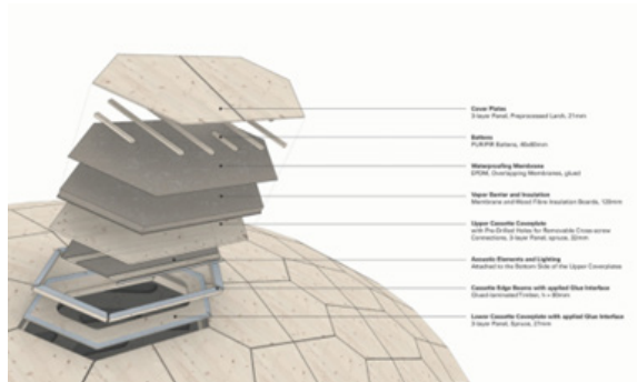
Figura 50. Esquema constructivo Pabellón 2023
