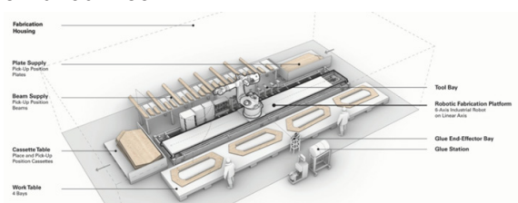
Figura 47. Robot colaborativo para Pabellón 2023
